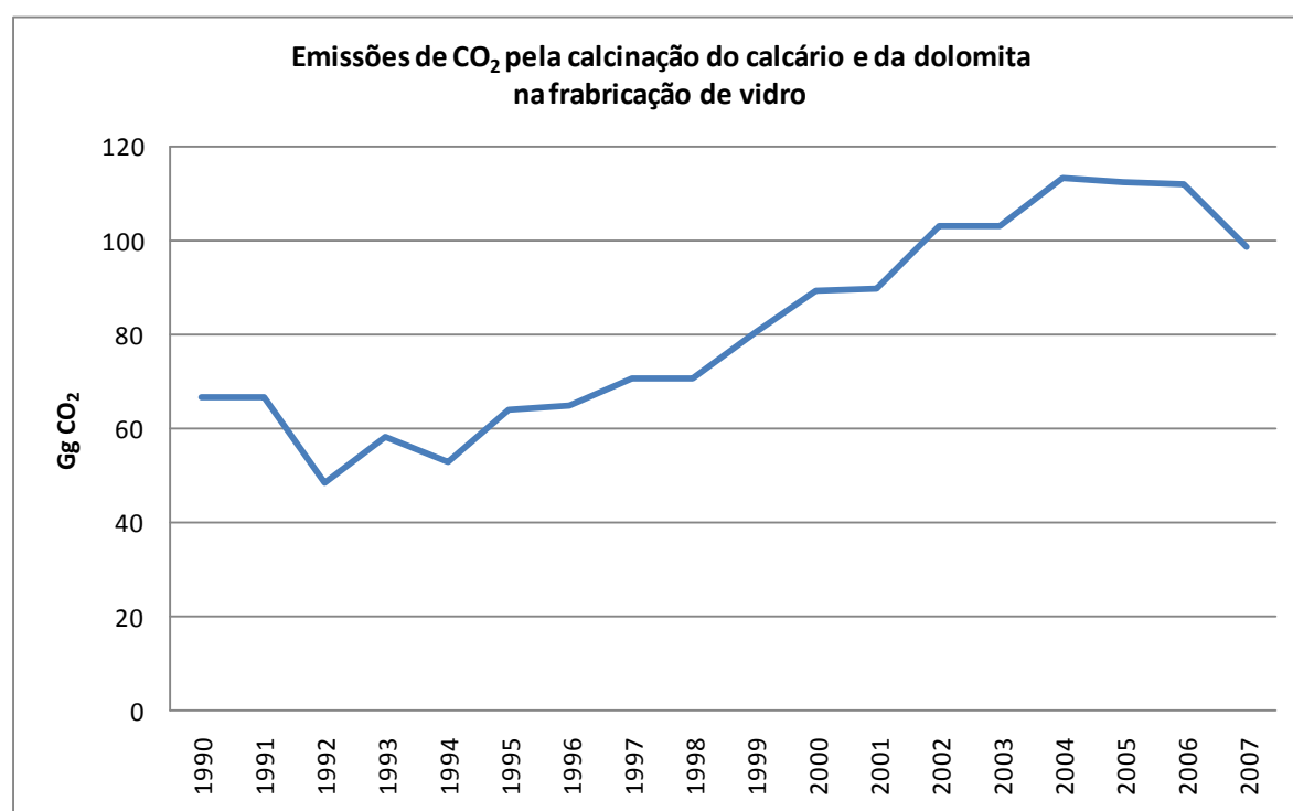
Figura 3 - Emissões de CO 2 na produção de vidro, de 1990 a 2007
