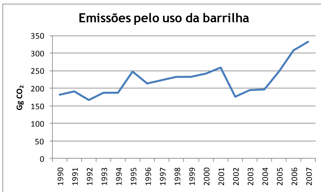
Figura 6 - Emissões de CO 2 pelo consumo da barrilha
