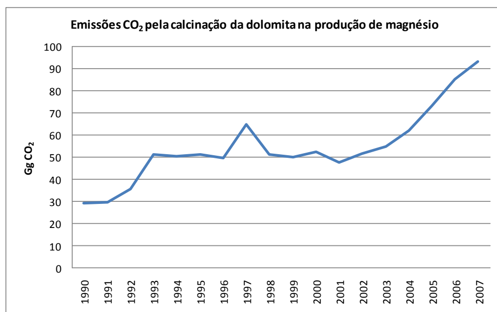
Figura 4 - Emissões de CO 2 pela calcinação da dolomita na produção de magnésio
