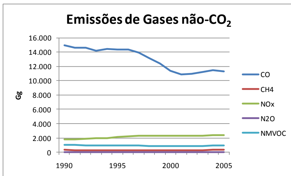
Figura II - Emissões de gases não- \text{CO}_2 devido à queima de combustíveis
