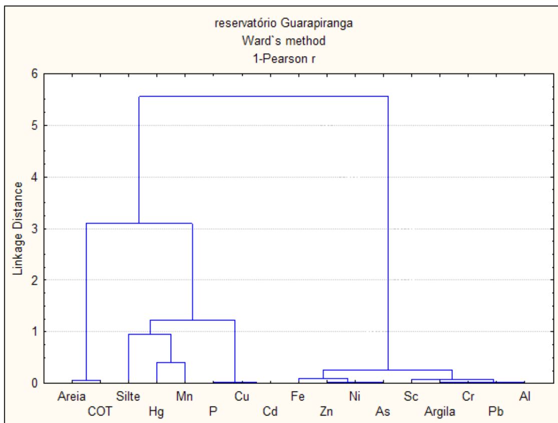
Figura 2 – Dendrograma obtido com os resultados do perfil do reservatório do Guarapiranga.
