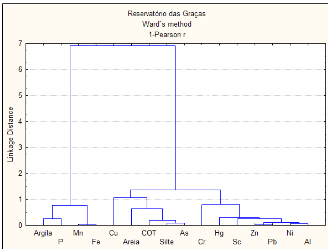
Figura 6 – Dendrograma dos parâmetros quantificados no perfil do reservatório das Graças.
