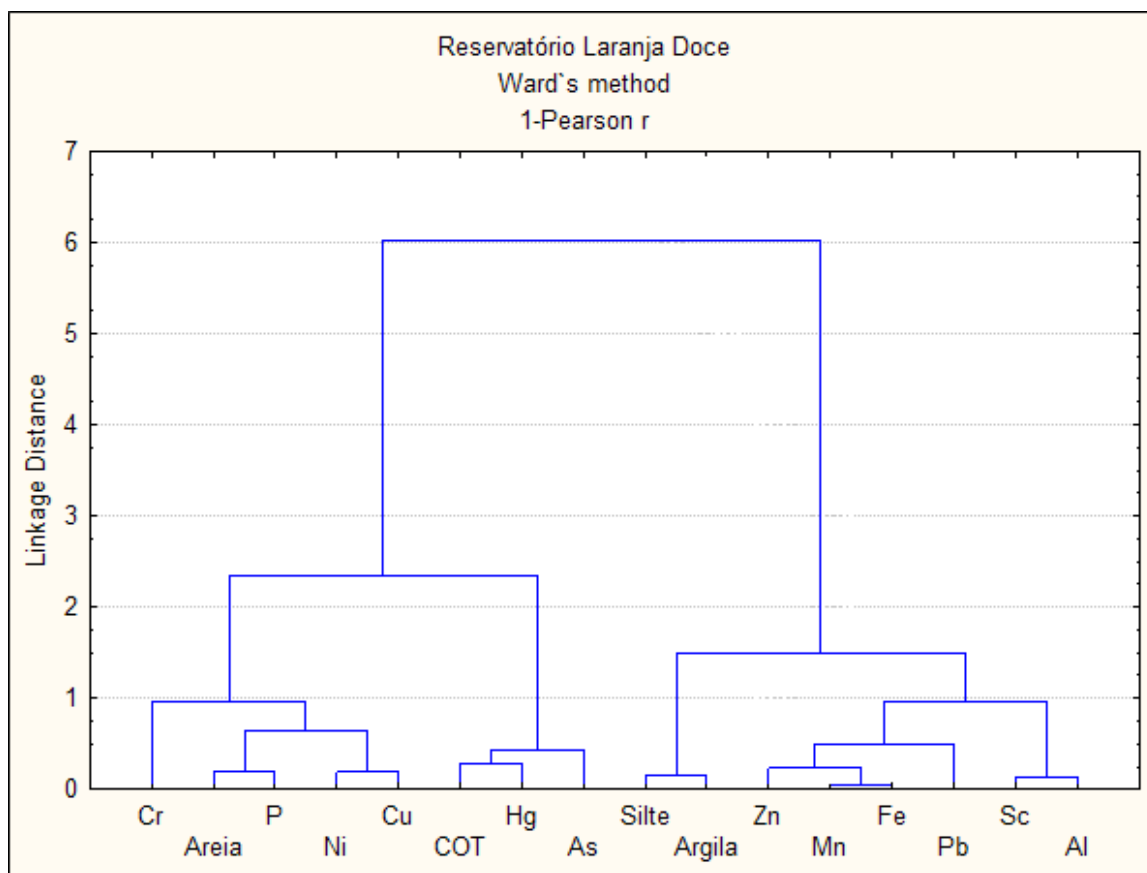
Figura 8 – Dendrograma obtido com as variáveis analisados no perfil sedimentar do reservatório da Laranja Doce.
