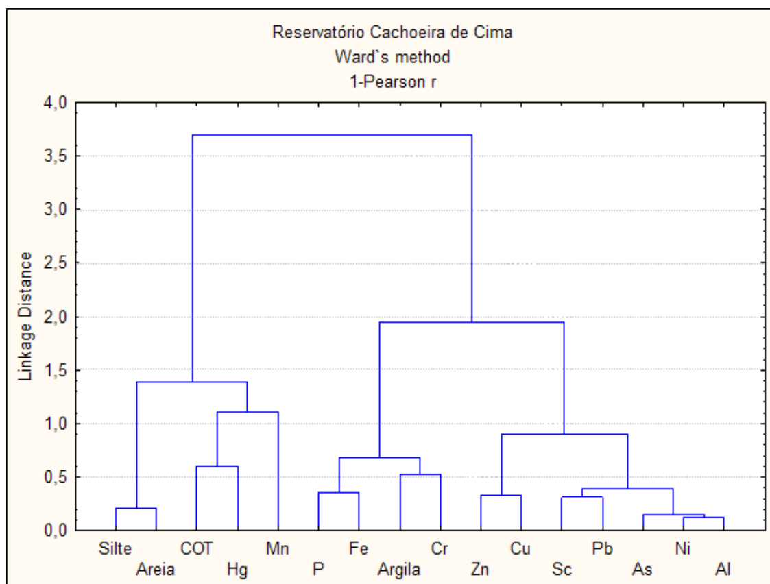
Figura 4 – Dendrograma obtido para o reservatório do Cachoeira de Cima com os elementos analisados.
