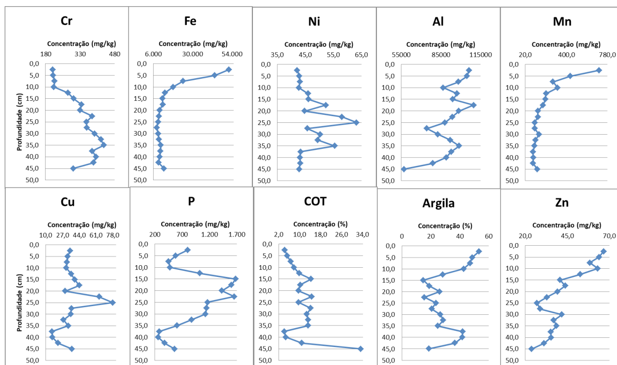
Figura 7 – Concentrações de alguns elementos, COT e argila ao longo do perfil do reservatório da Laranja Doce.
